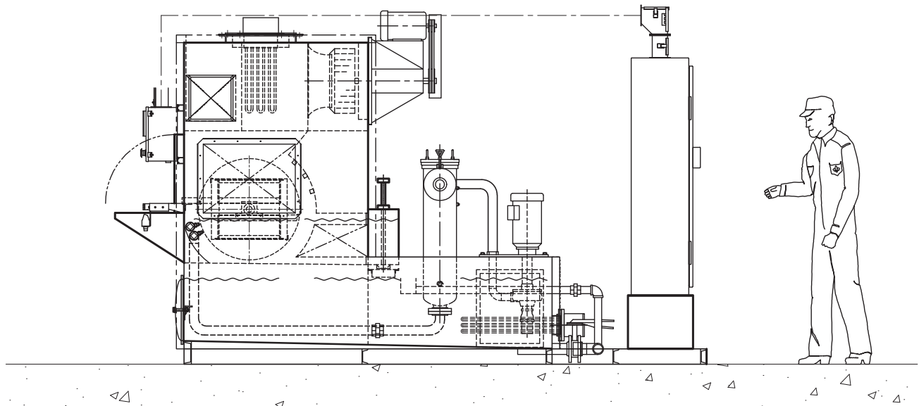
ELEVATION
